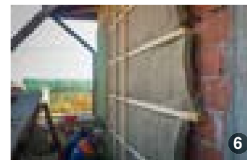
AȘA DA: Termoizolația din lână este deosebit de recomandată. Folosirea unei izolații din lână sprijină o industrie a prelucrării produselor locale: în mod frecvent, lâna se aruncă, în loc să fie utilizată. Această măsură este încă la început în țara noastră, dar se folosește cu succes și pe scară largă în majoritatea țărilor europene.
