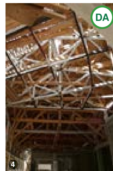
AȘA DA: Pentru construcții cu deschideri mari se pot folosi sisteme combinate de metal cu lemn.
