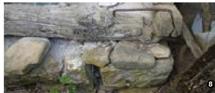
Fundație și soclu de piatră.
