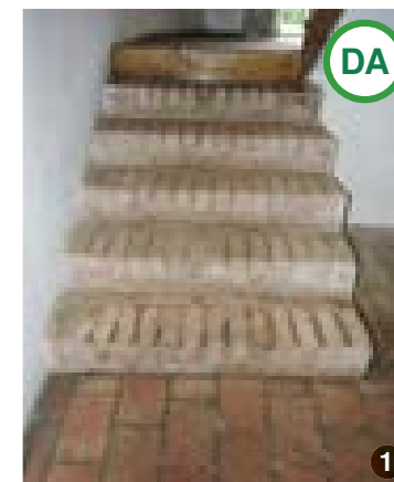
AȘA DA: Realizarea treptelor și a pardoseli din cărămidă.
