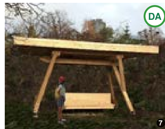
AȘA DA: Exemplu de construcție de protecție care poate fi folosită și la scară mai mare, pentru refugii și stație de autobuz.
