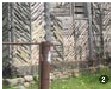
Perețe de lemn cu tencuială de lut pe șipci.
